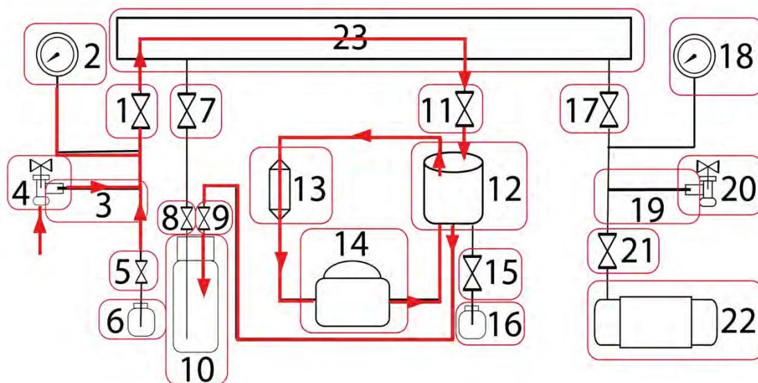
Схема 2. Заправка хладагентом внутреннего бака станции
