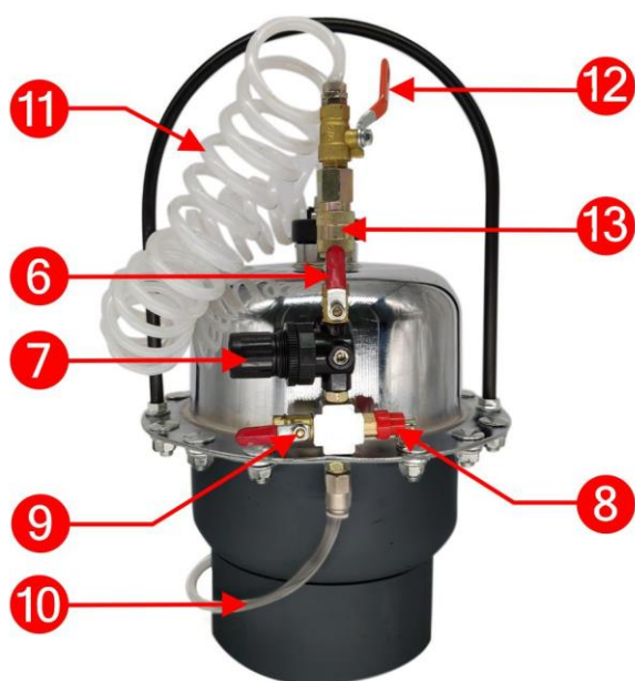
Рис.2 Устройство изделия
