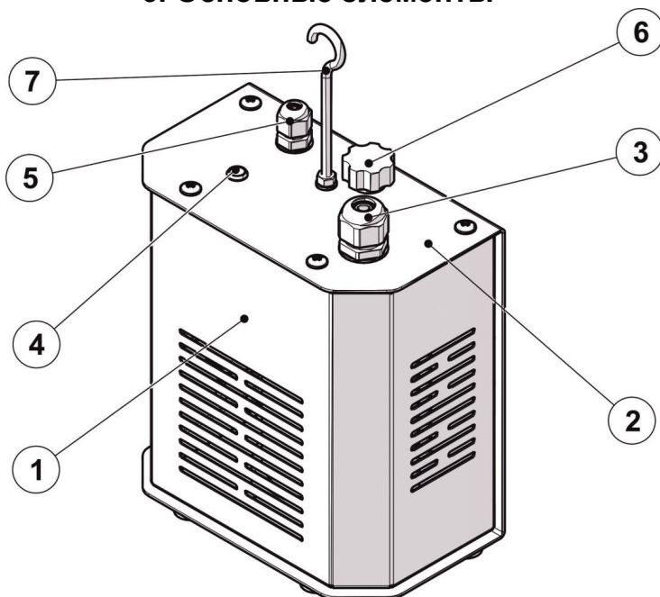
Рис. 3 Основные элементы дымогенератора
