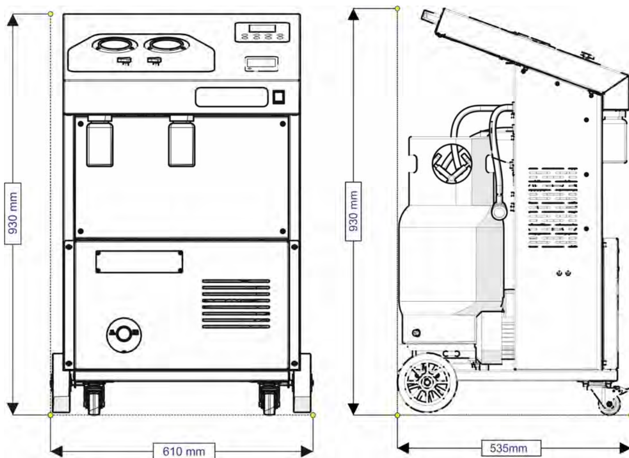
Рис. 1 Общй вид установки
