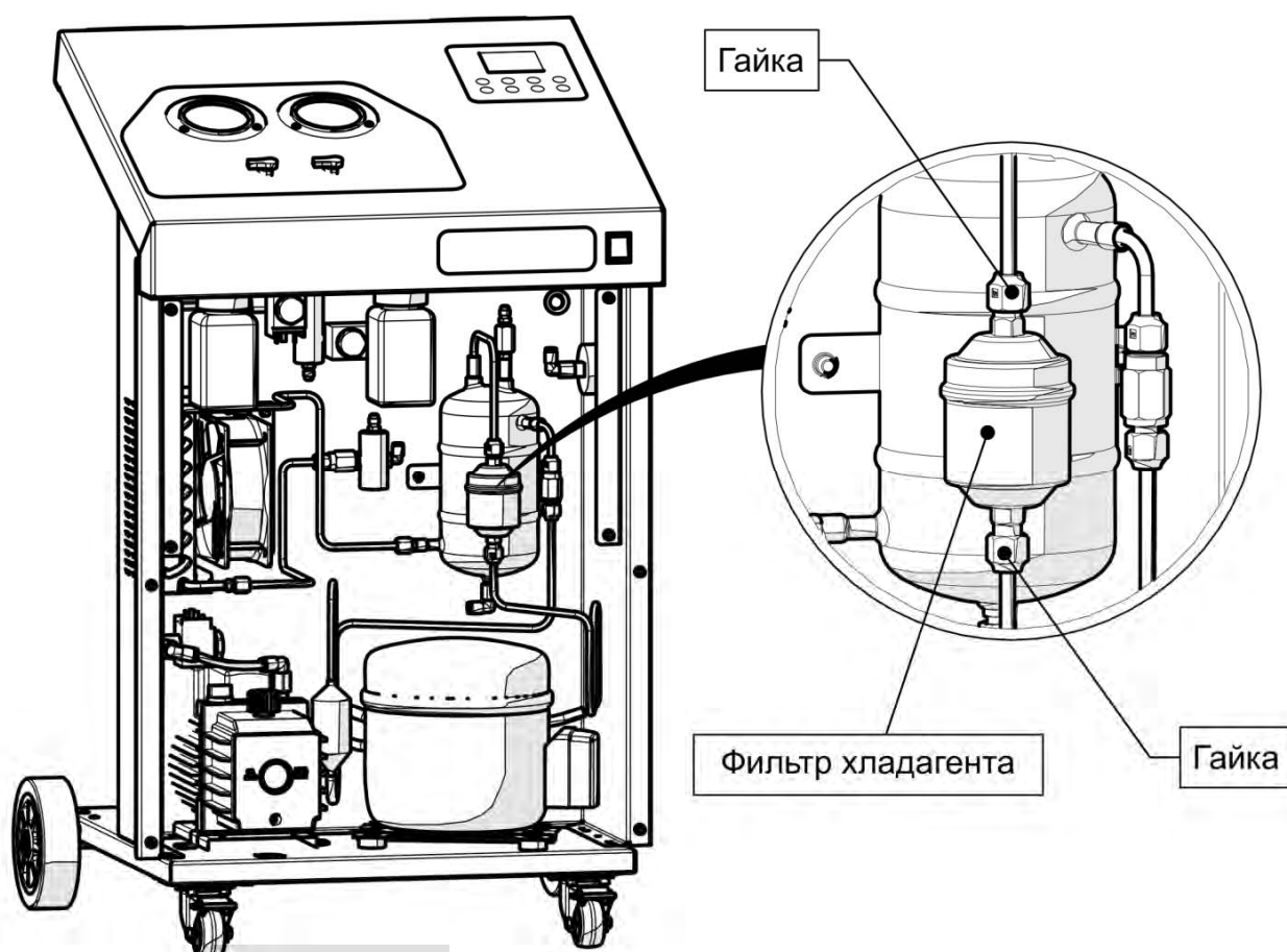
Рис. 10 Замена фильтра хладагента.
