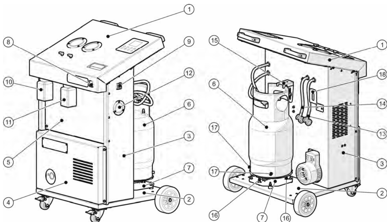
Рис. 2 Основные элементы станции ODA-360AP
