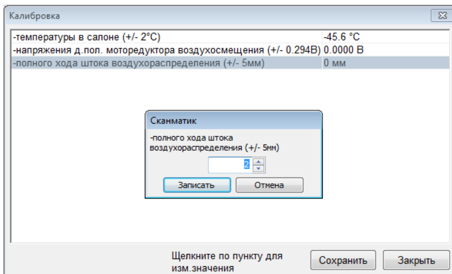
Конфигурация (калибровка)
