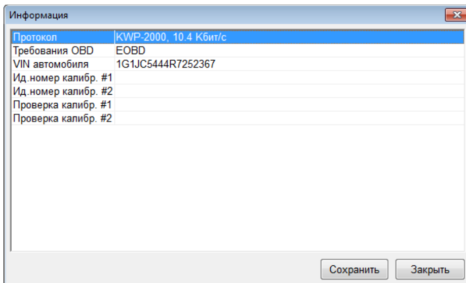
Режим "Информация".
