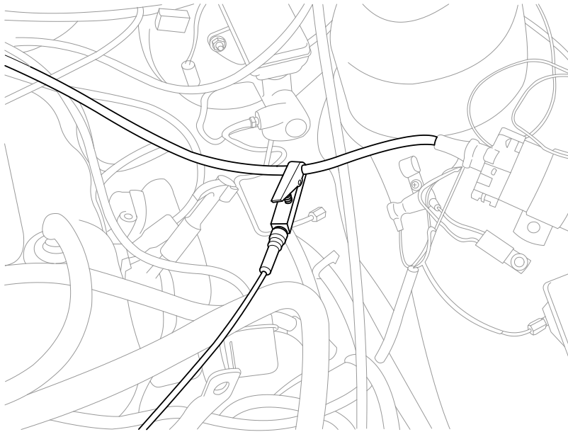
Подключение датчика вторичного напряжения центральному проводу
