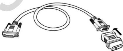
Рисунок 3-1. Подключение адаптера OBD II к главному кабелю с разъемом DB15
