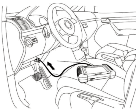
Рисунок 3-6. Подключение главного кабеля к диагностическому разъёму автомобиля.
